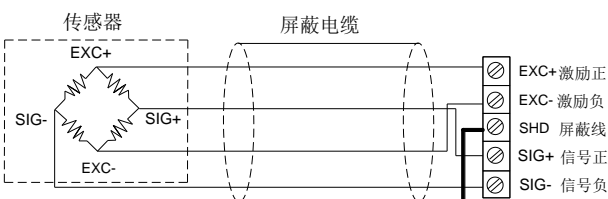
4芯传感器与仪表接线图
