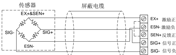
4芯传感器与仪表接线图
